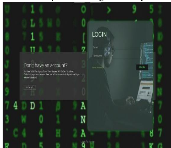
Fig.1.: Login Module
